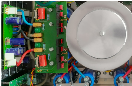
Ein Blick unter die Haube: Hier sehen wir den oberen der beiden übereinander gesetzten Mu-Metall-Transformatoren. Für die Anniversary Edition kommen extraprotekte Versionen zum Zuge: Jeder dieser Trrafos hat eine Lieferfähigkeit von 800 Voltampere - macht in Summe satte 1.600 Voltampere. Am unteren Rand sieht man die kleineren Elkos, die als Pufferung für die großen Elektrolytkondensatoren der Stromversorgung dienen. Ihre Verbindung über Metallschienen sorgt für eine bessere Energieabgabe. Ansonsten verwendet Symphonic Line zur Verbindung extrem hochwertiges Leitermaterial, das auch in den Signalkabeln der Manufaktur zum Einsatz kommt.
