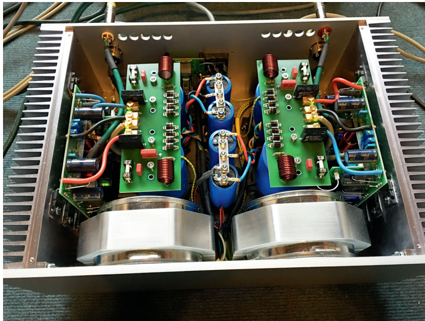
NEU 2023: Endverstärker RG 7 MK 5 Reference und Edition
