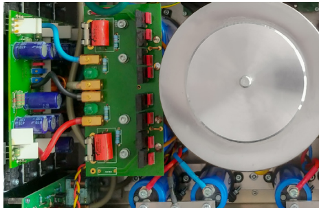
Ein Blick unter die Haube: Hier sehen wir den oberen der beiden übereinander gesetzten Mu-Metall-Transformatoren. Für die Anniversary Edition kommen extraprotierte Versionen zum Zuge: Jeder dieser Trrafos hat eine Lieferfähigkeit von 800 Voltampere - macht in Summe satte 1.600 Voltampere. Am unteren Rand sieht man die kleineren Elkos, die als Pufferung für die großen Elektrolytkondensatoren der Stromversorgung dienen. Ihre Verbindung über Metallschienen sorgt für eine bessere Energieabgabe. Ansonsten verwendet Symphonic Line zur Verbindung extrem hochwertiges Leitermaterial, das auch in den Signalkabeln der Manufaktur zum Einsatz kommt.
